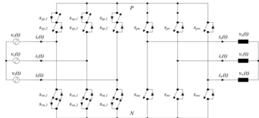
Figura 2 – Topologia do conversor matricial indireto.
