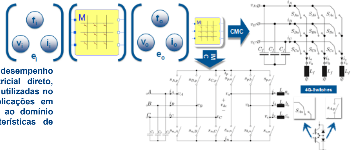
Figura 2 – Topologia do conversor matricial indireto.
